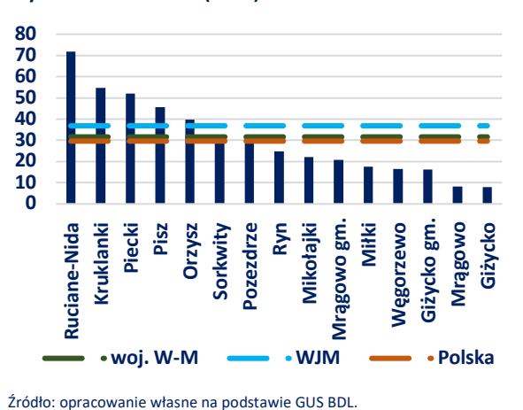
Wykres 5. Lesistość % (2018)
